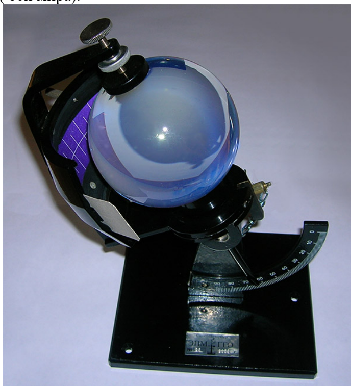
Рис. 5. Универсальный гелиограф
