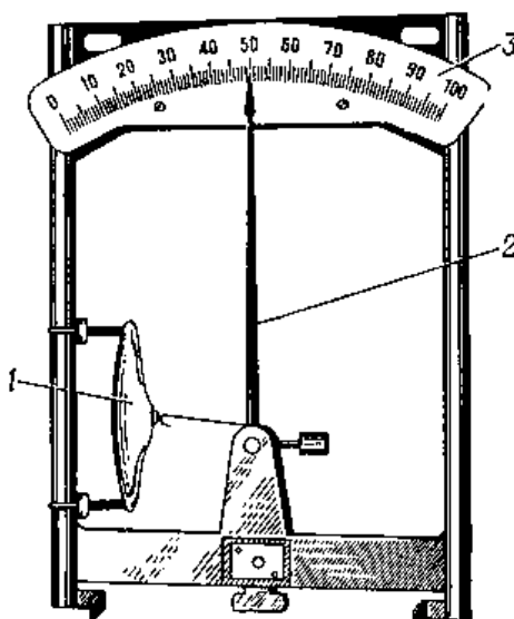
Рисунок 14. Пленочный гигрометр: 1 – пленка, 2 – стрелка, 3 - шкала
